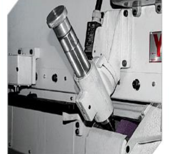
Taş bileme aparatı Grinding wheel dressing apparatus
